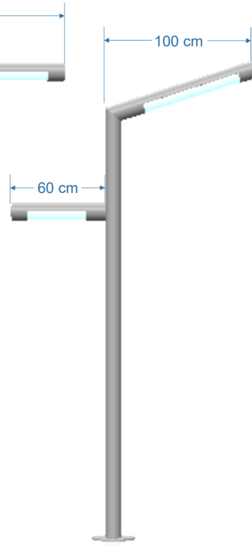
EL-98.1447 h:350 cm Çelik Boru 36W Led
