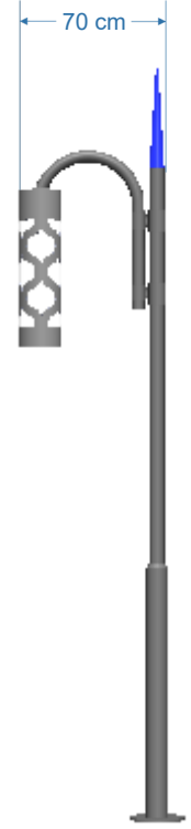
EL-98.1443 h:350 cm Çelik Boru 36W Led
